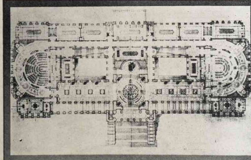
Distribución de la planta baja del "Capitolio Nacional", cuyas obras de construcción empezarán próximamente.
